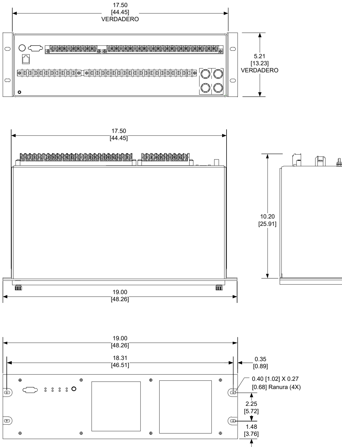
Estandar 19" Bastidor para Montage Horizontal
