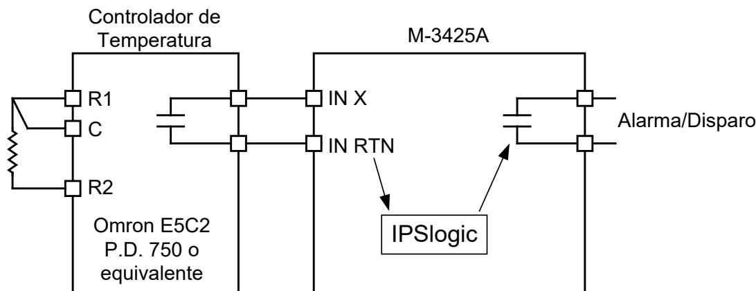
Figura 1 Aplicación Típica de Monitoreo del Controlador de Temperatura
