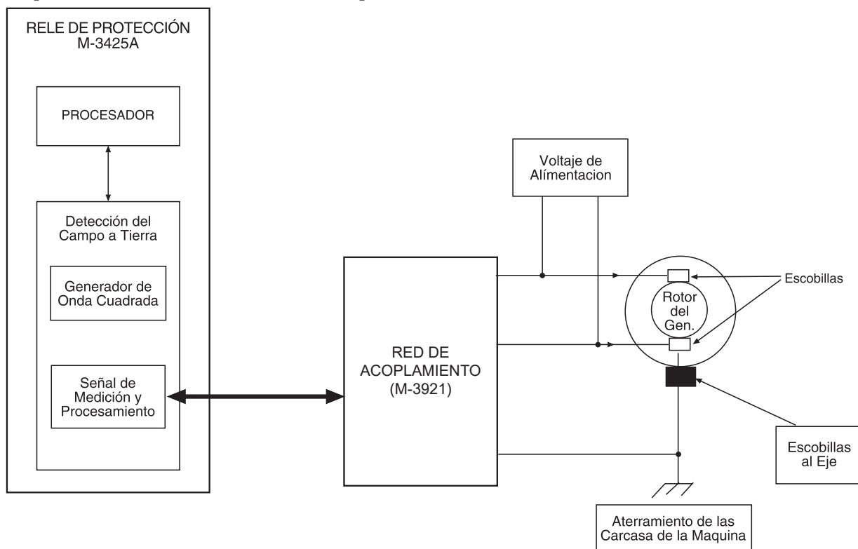
Figura 11 Diagrama de Bloque Protección del Campo a Tierra
