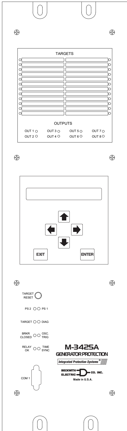
Figura 8 M-3425A Vertical de la Unidad Disposición
