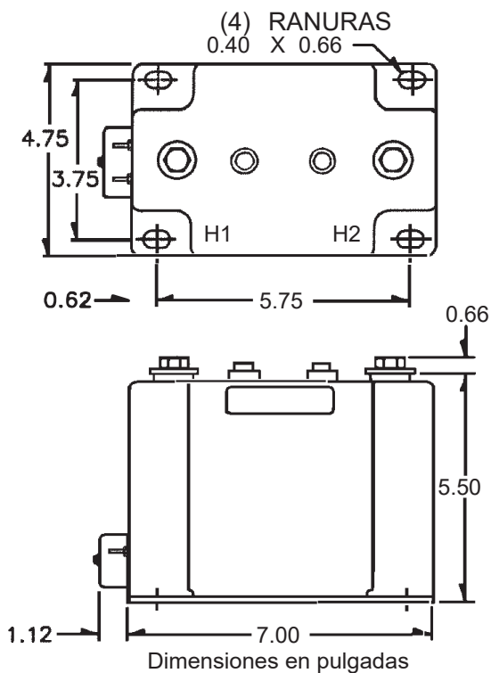
Figura 17 Transformador de Medición de Corriente de 20 Hz TC 400-5 A TC
