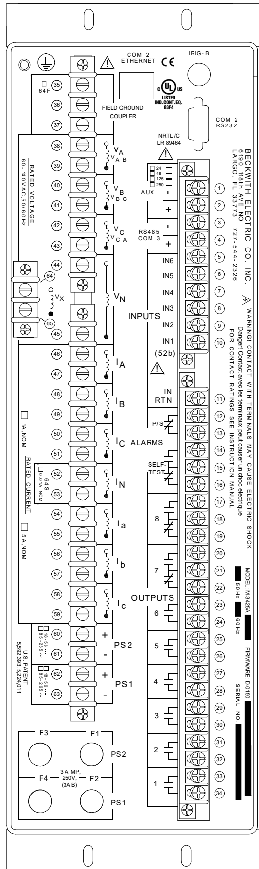
Figura 8 M-3425A Vertical de la Unidad Disposición
