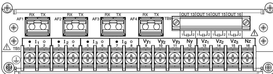
Figura 3 M-7651A Conexiones Externas (Módulo de Arco Eléctrico Opcional)
