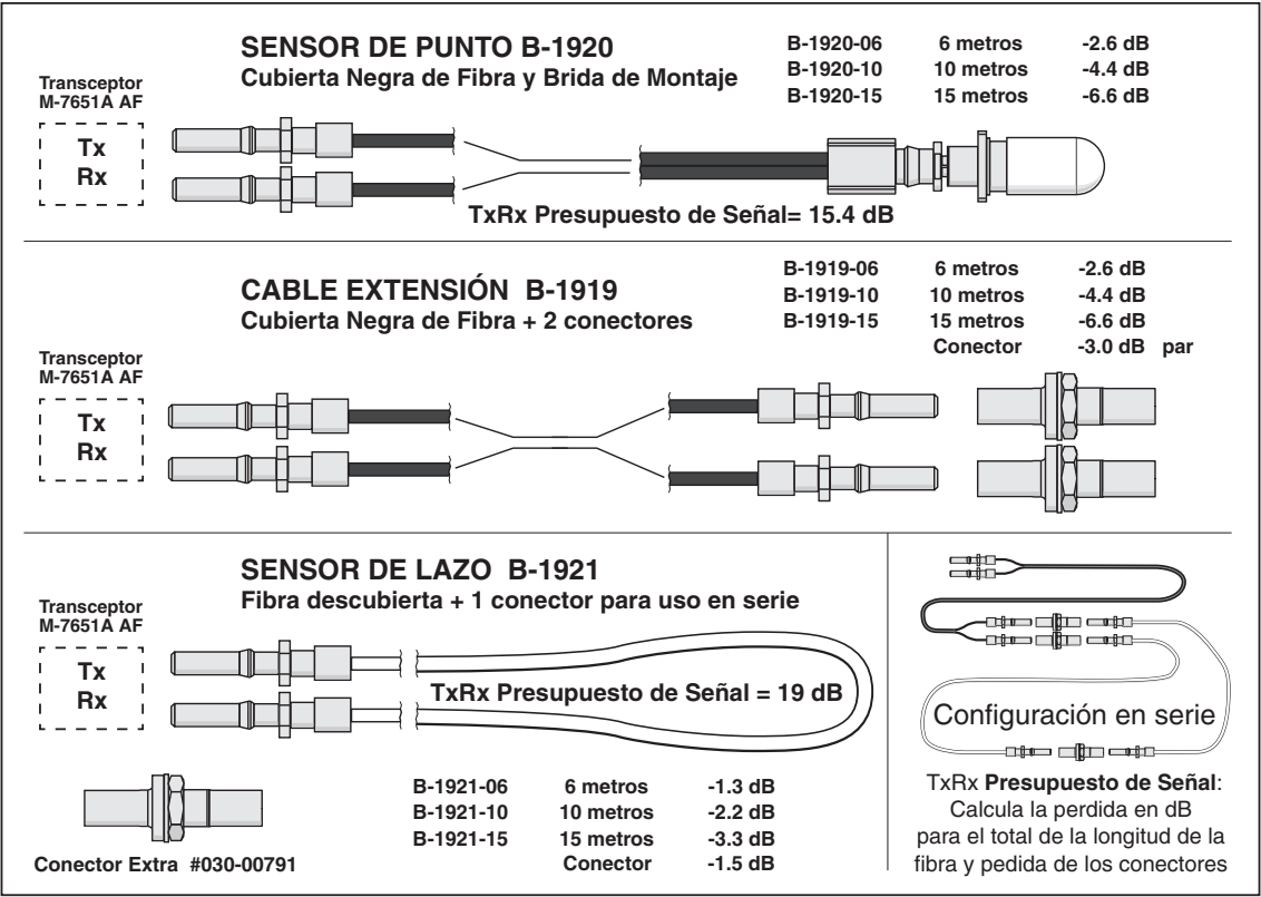
Figura 4 Opciones de Configuración del Sensor de Bucle y Sensor de Punto
