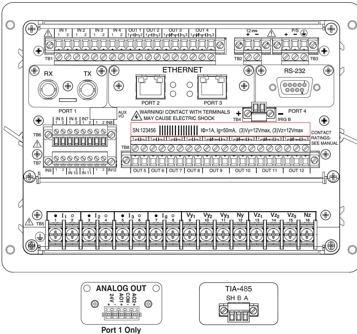
Figura 2 Conexiones externas del M 7651A (configuración típica, otras opciones disponibles)
