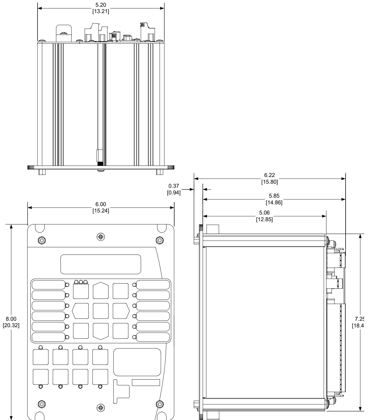
Figura 11 M-7651A D-PAC Dimensiones de Montaje del Modelo Vertical
