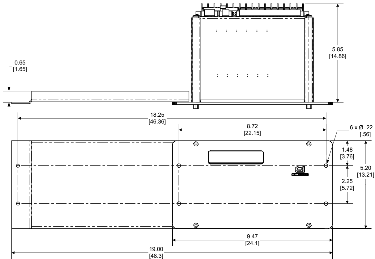
Figura 12 Dimensiones del bastidor del adaptador de montaje en bastidor de 19 pulgadas M-7651A D-PAC
