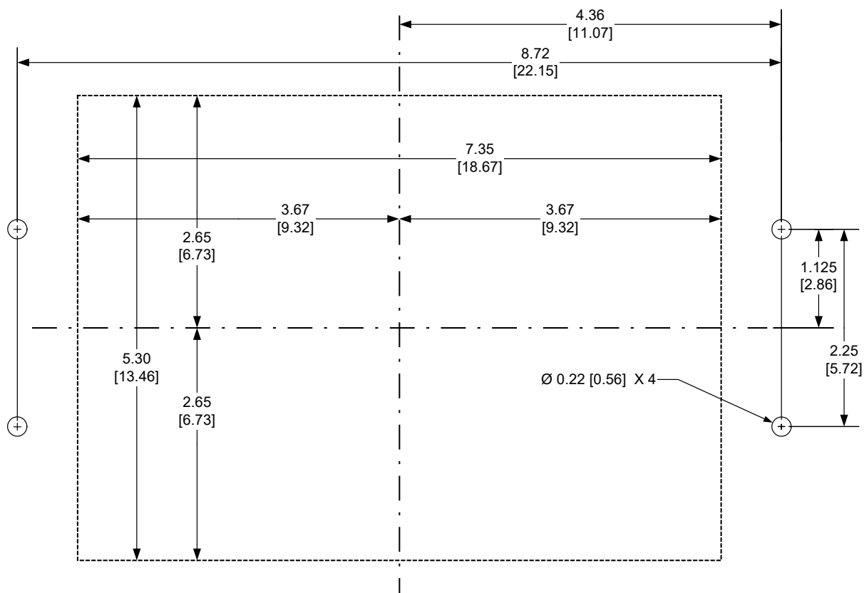
Figura 13 Dimensiones de corte para montaje en panel horizontal
