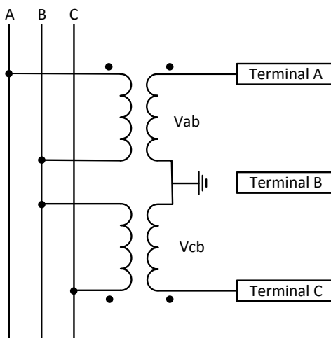
Figura 8 Diagrama Ejemplo de Delta Abierta CA
