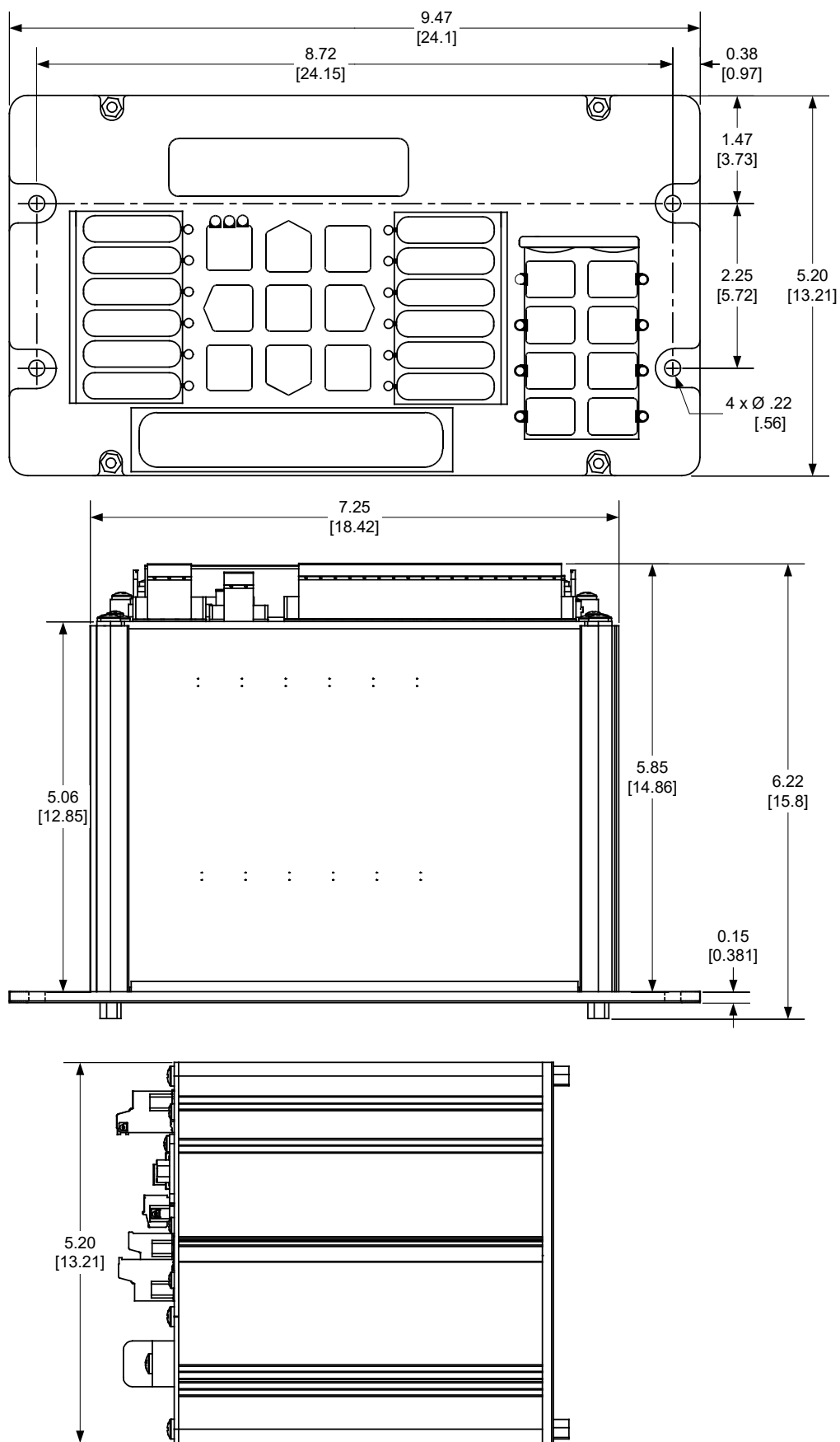
Figura 10 M-7651A D-PAC Dimensiones de Montaje del Modelo Horizontal
