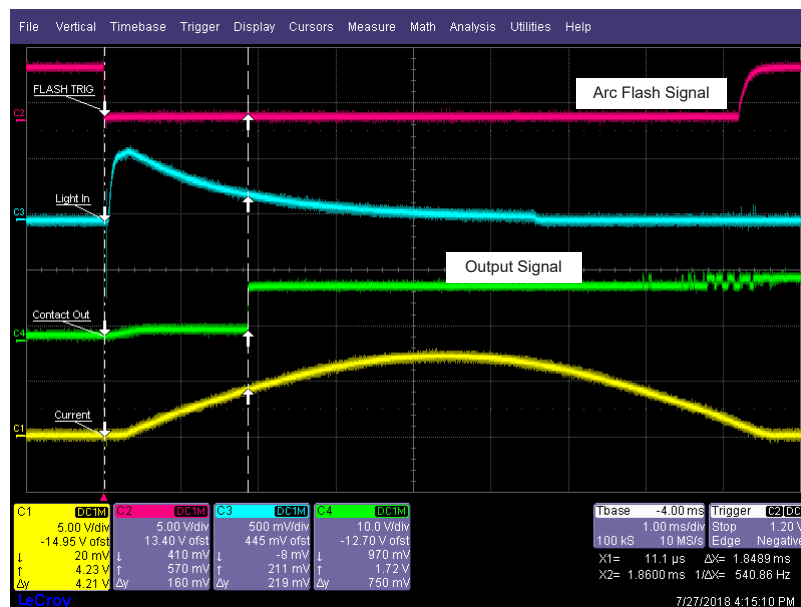
Figura 6 Ejemplo de Velocidad de Disparo de Salidas de Arco eléctrico (flash a 0 ° de 5 A actual – \Delta t = 1.85 ms)
