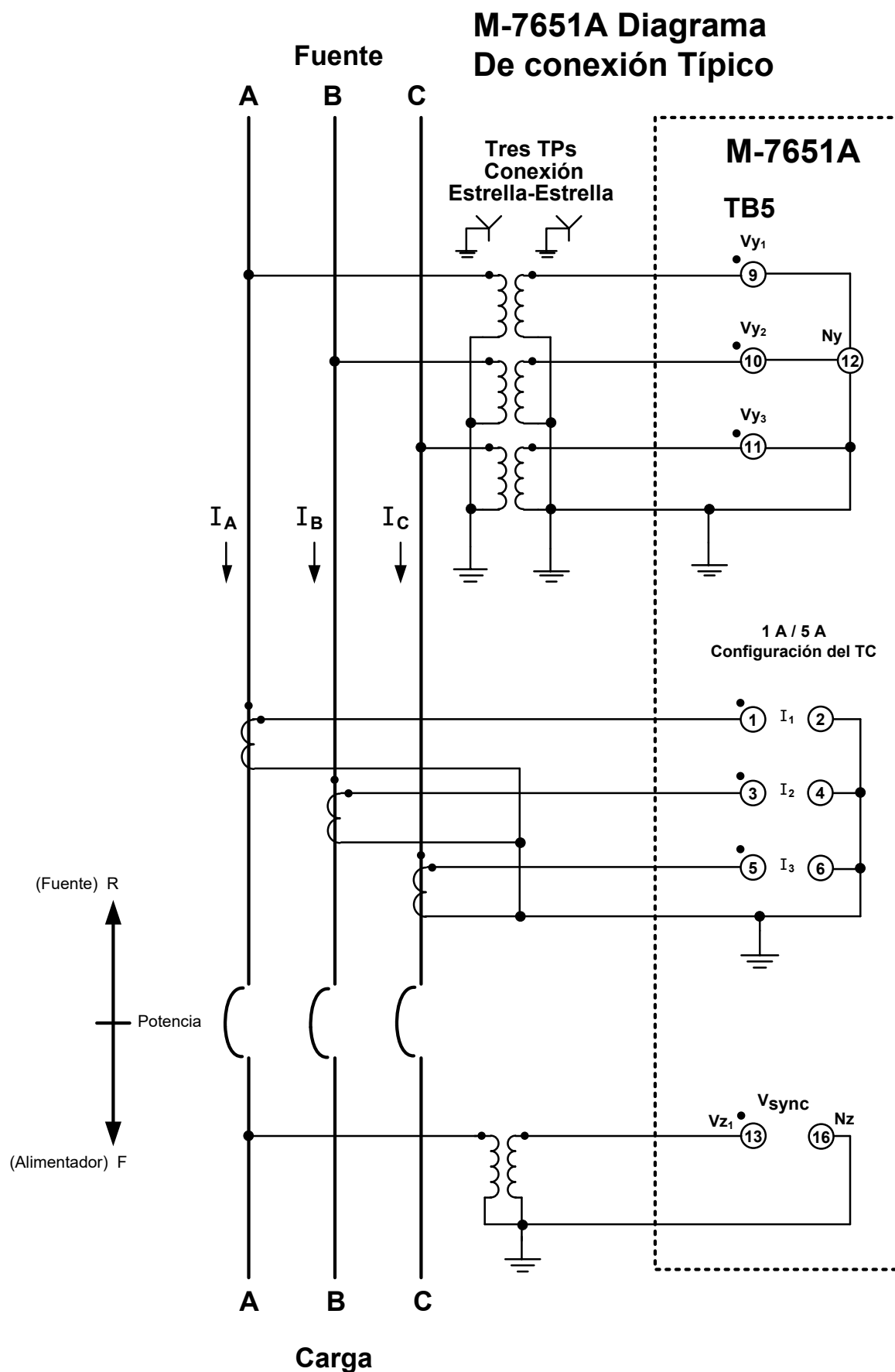
Figura 9 Diagrama de Conexión de Tres Líneas M-7651A D-PAC
