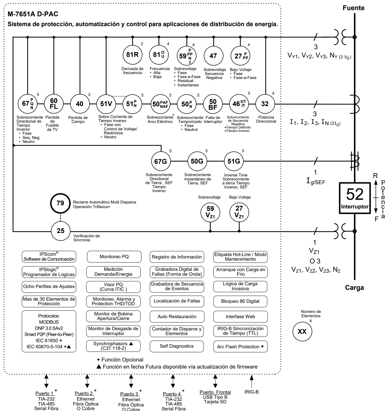
Figura 1 Diagrama unifilar funcional del M-7651A D-PAC
