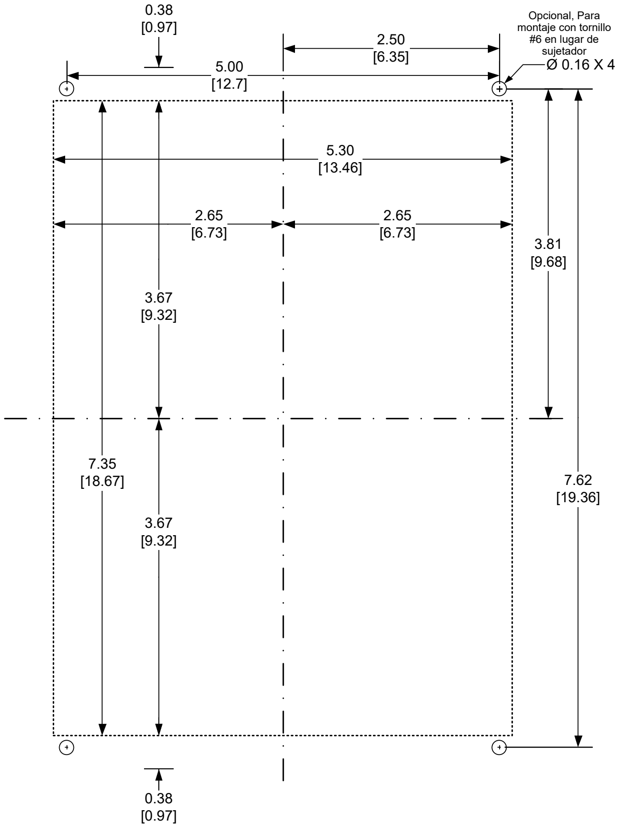
Figura 14 Dimensiones de corte para montaje en panel vertical
