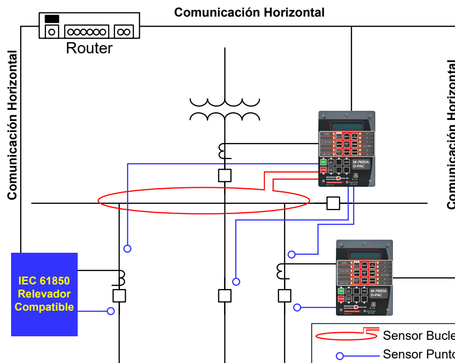
Figura 5 Diagrama de Comunicaciones Adicional del módulo de arco eléctrico M-7651A
