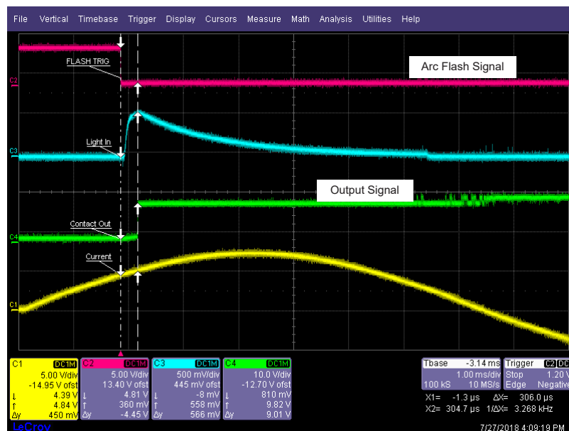
Figura 7 Ejemplo de Velocidad de Disparo de Salidas de Arco eléctrico (flash a 45 ° de 5 A de corriente – \Delta t = 306 \mu s)
